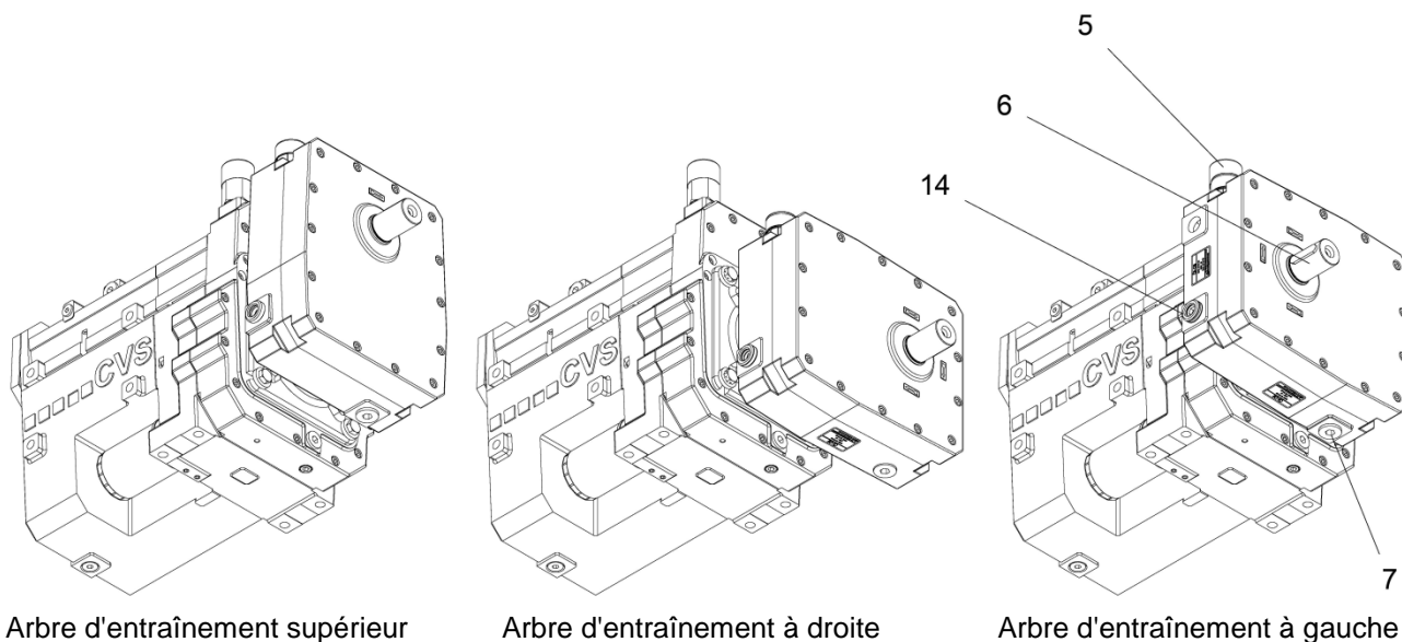
Fig. 2 : Vue du SiloKing de type LS avec réducteur à engrenages
