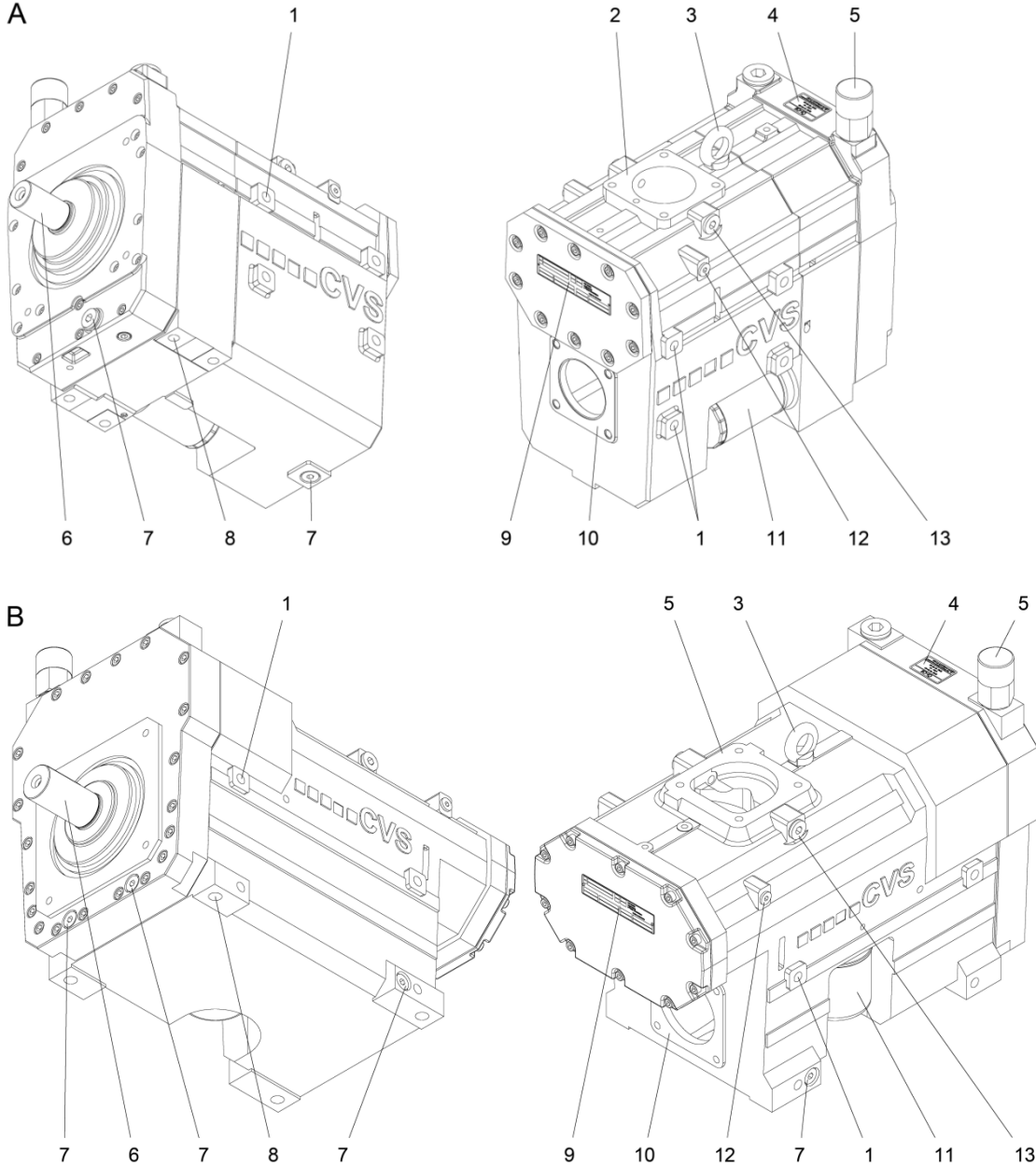
Fig. 1 : Vue du SiloKing et détails
